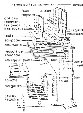
SCHEMA DU MECANISME DE L'ORGUE
